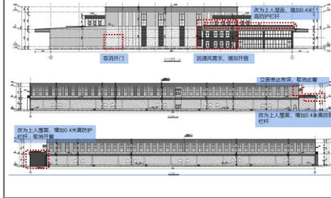
1-2#变更后立面图
