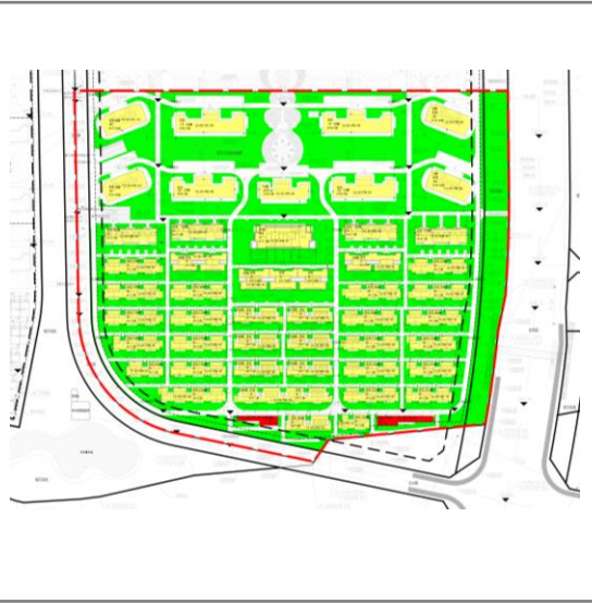
变更后总平面图
