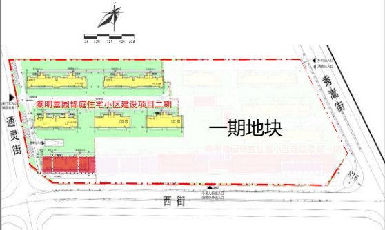
总平面图
