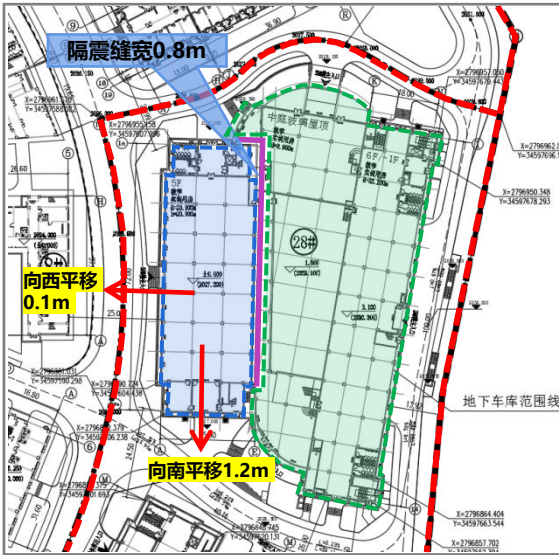
变更后总平面图
